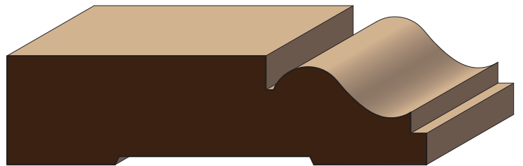
CA 472 13/16 x 3 1/8
